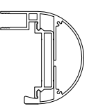
8 LRT 101 1 : 5
