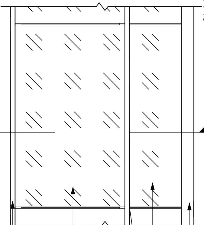
1 Plan 1 : 15
