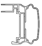
10 LRT 103 1 : 5
