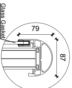
4 Detail 1 1 : 5
