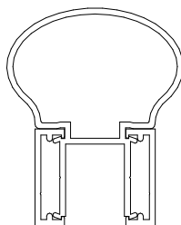
4 Top rail 1B 1:2
