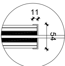
4 Detail 1 1 : 5
