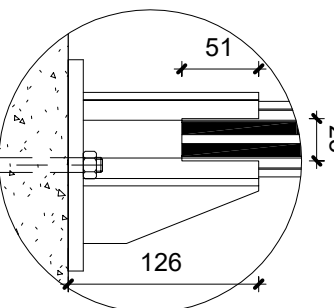
5 Detail 2 1 : 5
