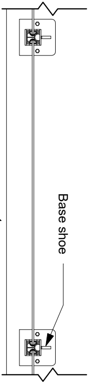
1 Plan 1 : 15
