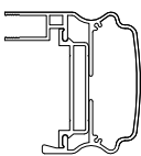
5 Detail 2 1 : 5
