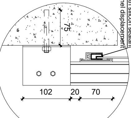
5 Detail 2 1 : 5
