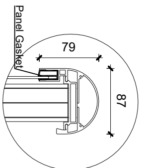
4 Detail 1 1 : 5
