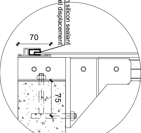
4 Detail 1 1 : 5
