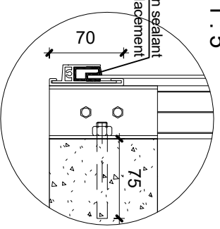
3 Detail 2 1 : 5
