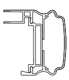
8 LRT103 1 : 5
