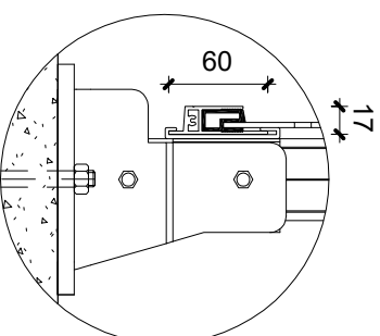
5 Detail 2 1 : 5
