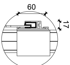
4 Detail 1 1 : 5
