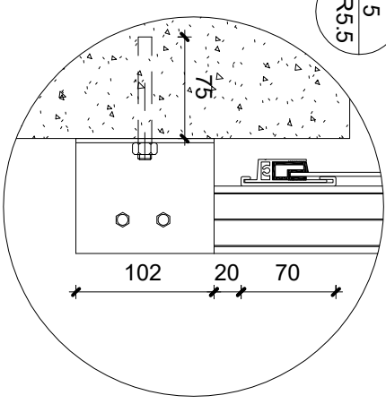
5 1 : 5
