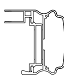
9 LRT103 1 : 5
