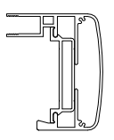
8 LRT102 1 : 5
