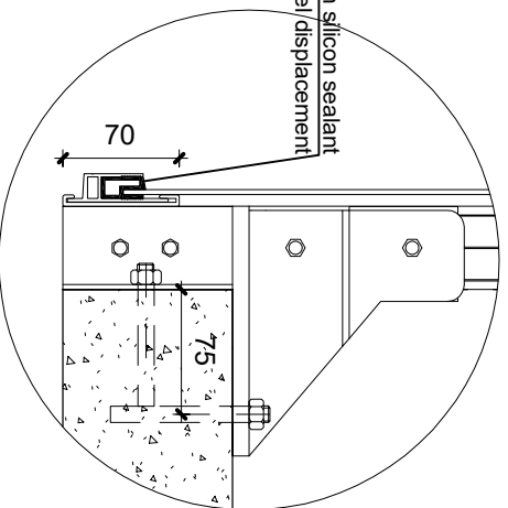
4 Detail 1 1 : 5
