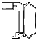
8 LRT103 1 : 5
