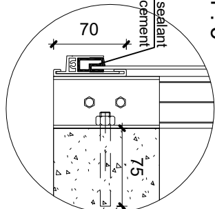
2 Detail 1 1 : 5
