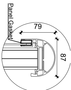
2 Detail 1 1 : 5
