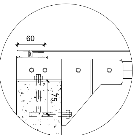
6 Detail 3 1 : 5
