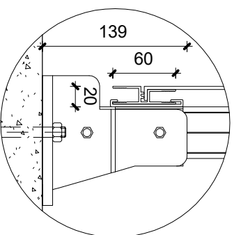
5 Detail 2 1 : 5
