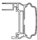
6 Detail 3 1 : 5
