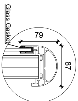
4 Detail 1 1 : 5
