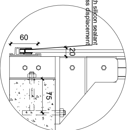
5 Detail 2 1 : 5
