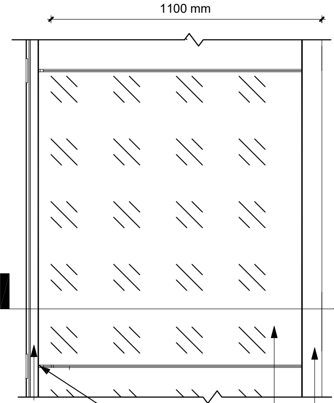
1 Plan 1 : 15
