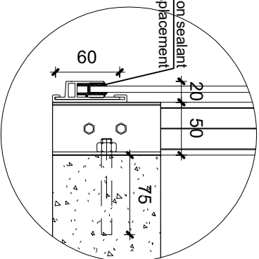
5 Detail 2 1 : 5
