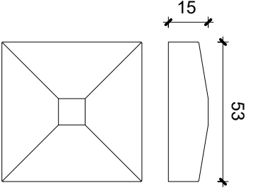
8 Top cap 1 1:2
