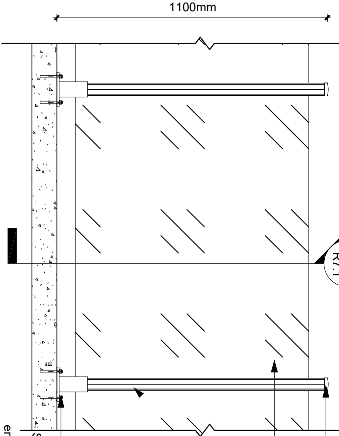
1 Plan 1:15
