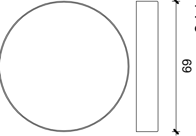
11 Top cap 4 1:2
