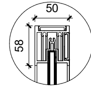
⑦ Detail 1 1 : 5
