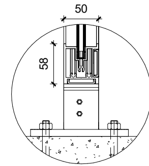
⑧ Detail 3 1 : 5
