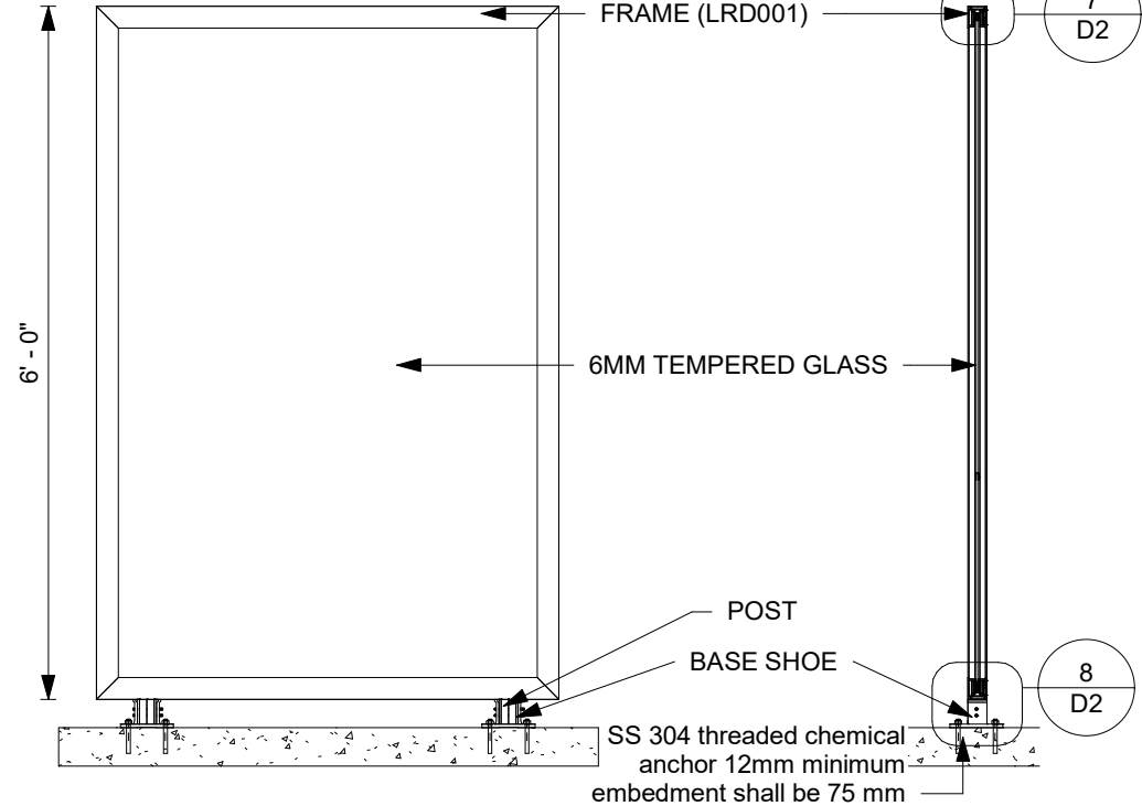
② Elevation 1 : 20
