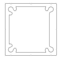
4 LRP001 1 : 2
