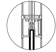
7 Detail 1 1 : 5
