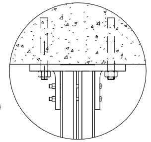
9 Detail 3 1 : 5
