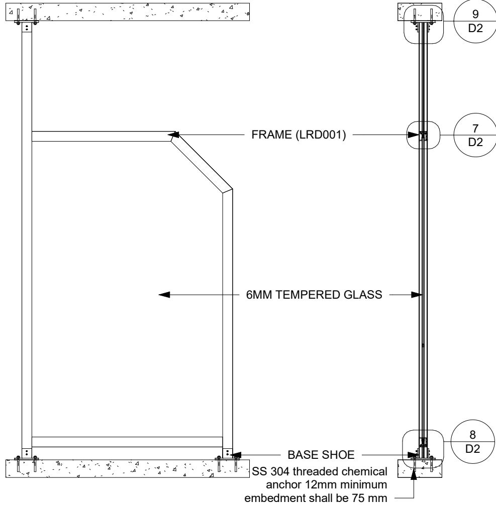
2 Elevation 1 : 20
