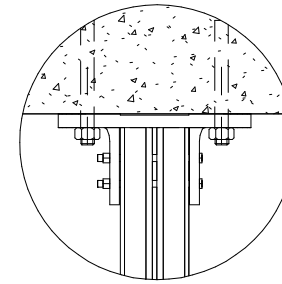
9 Detail 1 1 : 5
