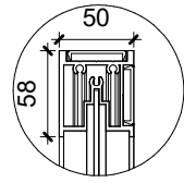
7 Detail 1 1 : 5
