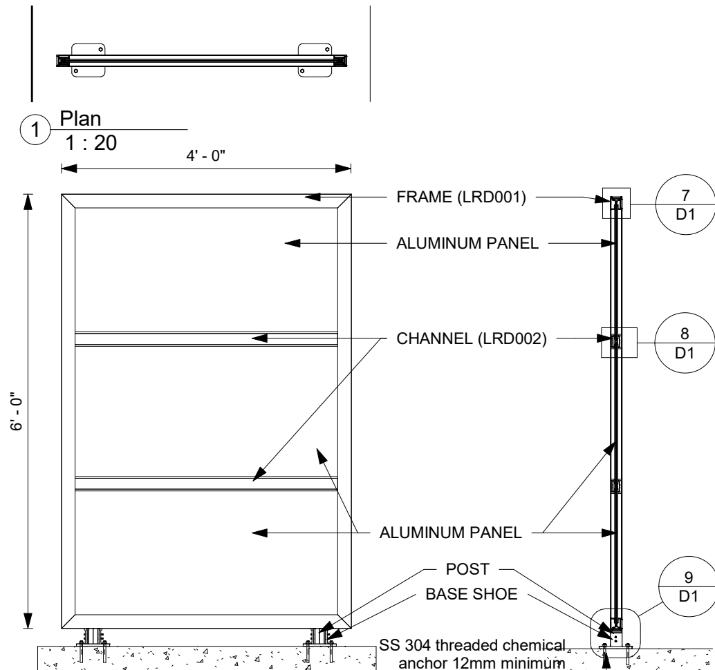
2 Elevation divider 1 : 20
