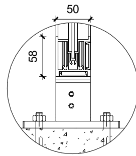
9 Detail 3 1 : 5
