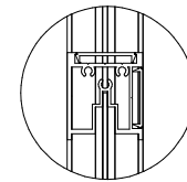
7 Detail 1 1 : 5
