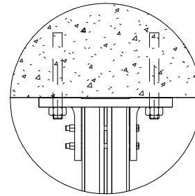
10 Detail 4 1 : 5
