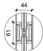
8 Detail 2 1 : 5
