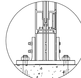
9 Detail 3 1 : 5
