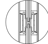
8 Detail 2 1 : 5
