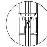
7 Detail 1 1 : 5
