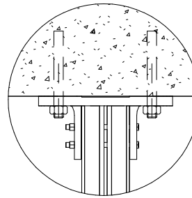
10 Detail 4 1 : 5
