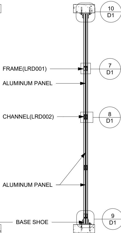
3 Cross section 1 : 20
