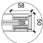
6 Detail 1 1 : 5
