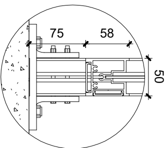
8 Detail 3 1 : 5
