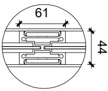
7 Detail 2 1 : 5
