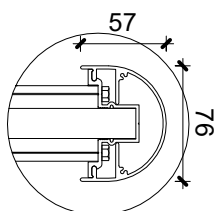
4 Detail 1 1 : 5
