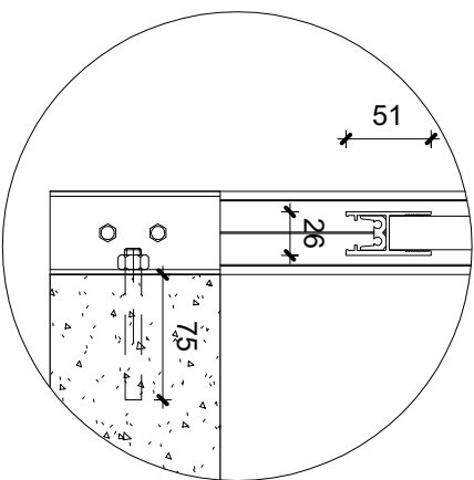
4 Detail 1 1 : 5
