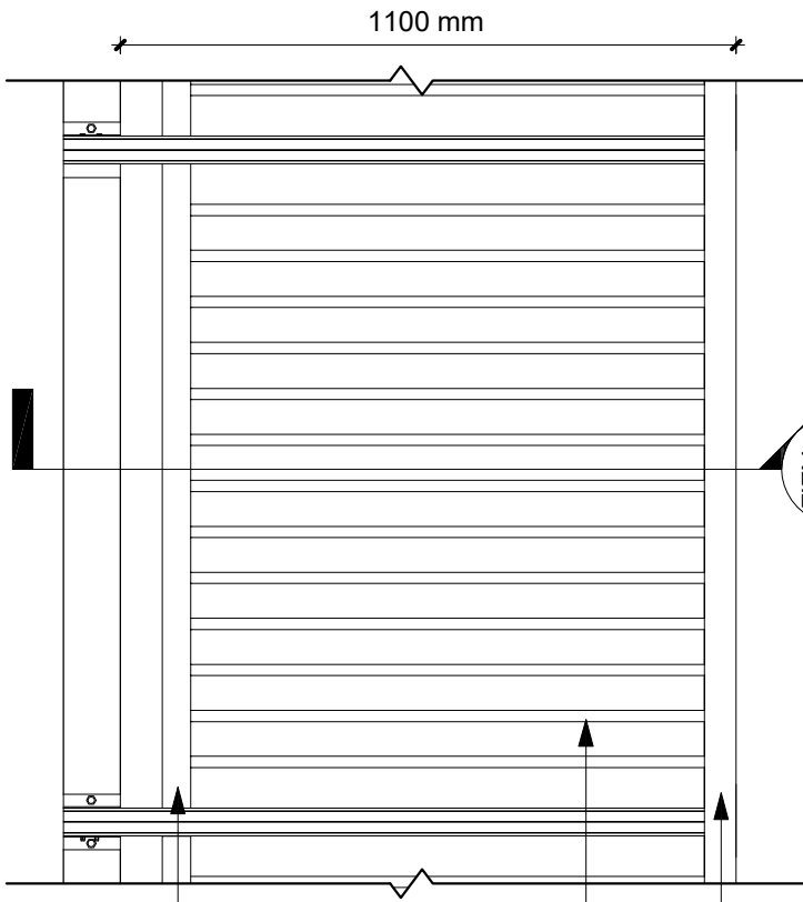
1 Plan 1 : 15
