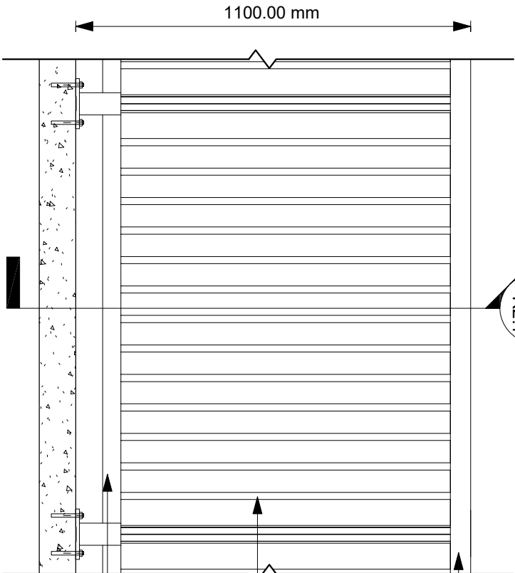
1 Plan 1 : 15
