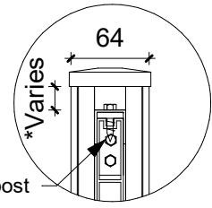
4 Detail 1 1 : 5
