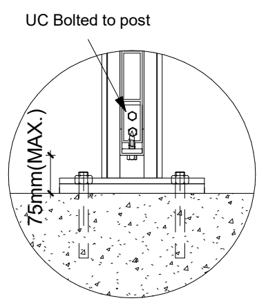
5 Detail 2 1 : 5
